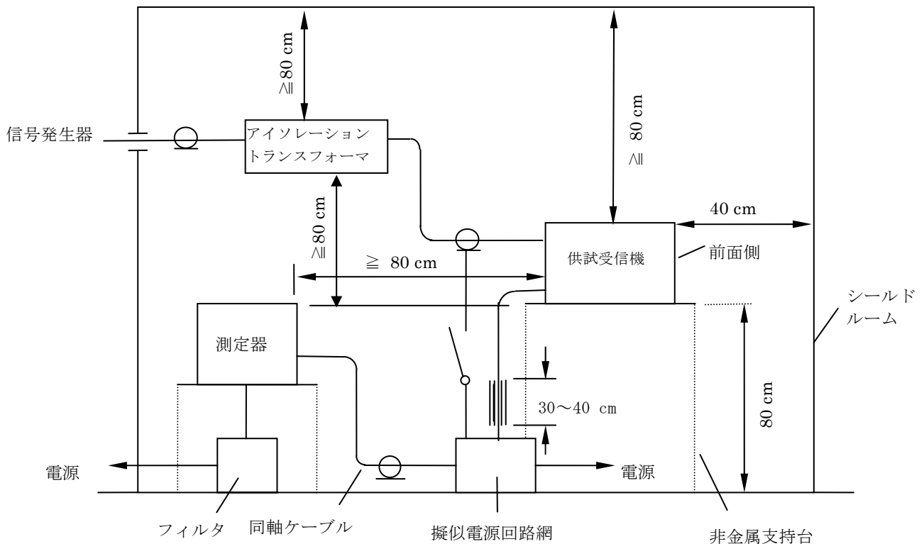
図A.1 150 kHz ～ 30 MHzの電源端子妨害波電圧測定（側面図）
