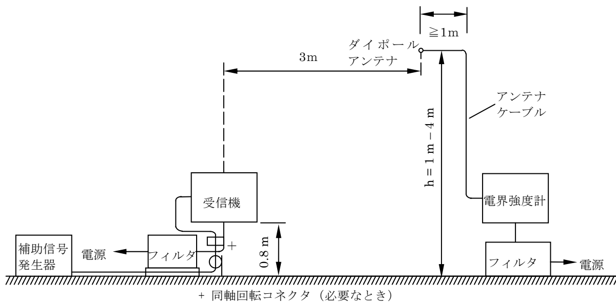
図 14 3 m の距離における屋外電界測定 (5.7.3 項参照)
